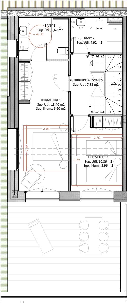
PLANTA PRIMERA
